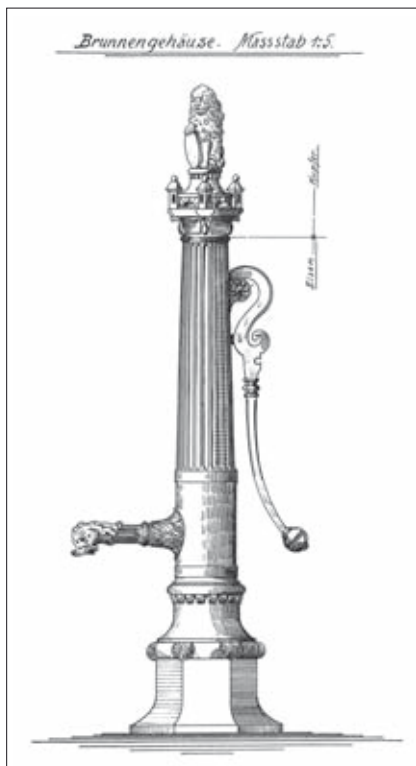
Entwurfszeichnung der Pumpe „Kleiner Löwe“ von 1908
