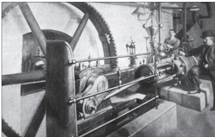
Dampfmaschine (70 PS), „Pura“, Wittenberger Straße 38, um 1907
